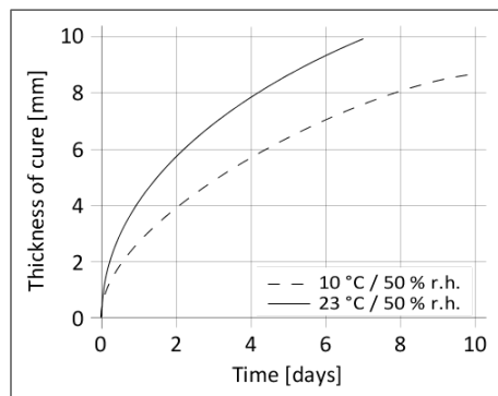
Diagrama 1: Velocidad de curado para Sikaflex®-221
